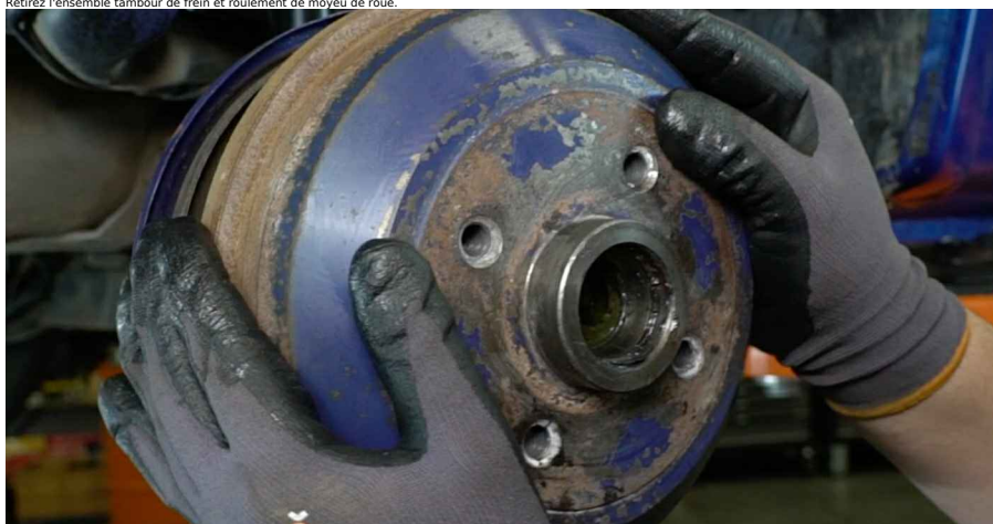
Remplacement : roulement de roue - VAUXHALL CHEVETTE. Conseil d'AUTODOC :
