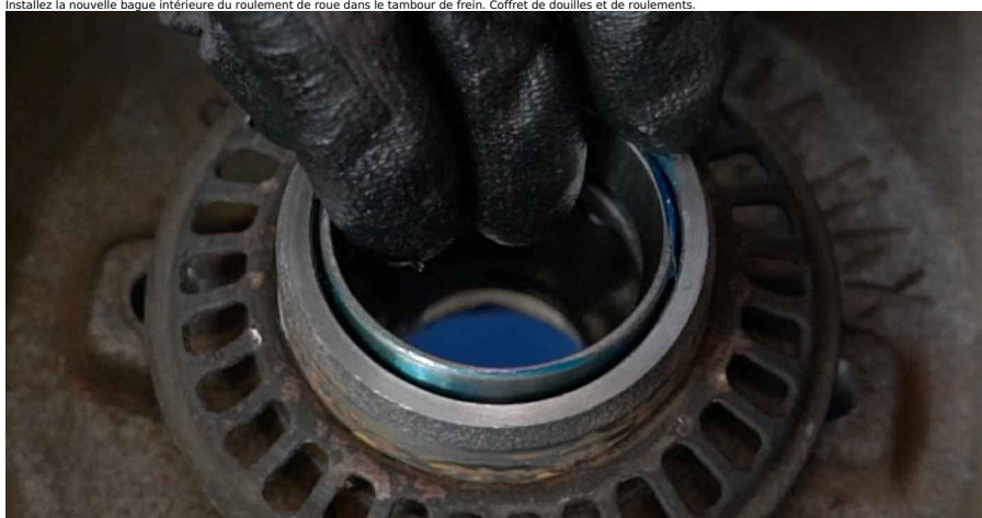
20 Appliquez du produit sur le palier de moyeu de roue. Utilisez de la graisse pour roulements.
