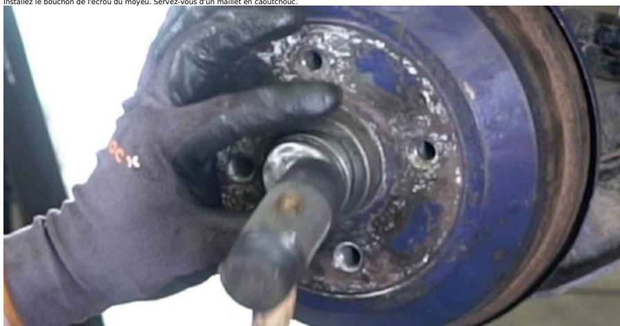
35 Appliquez du produit sur la surface de contact entre la jante et le tambour de frein. Utilisez du lubrifiant céramique.
