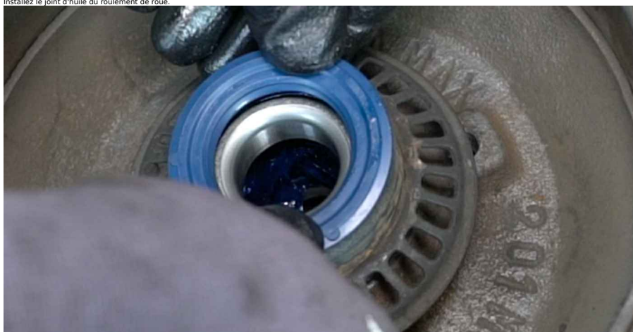
23 Appliquez du produit sur la fusée d'essieu. Servez-vous d'un aérosol nettoyant multi-usages. Utilisez de la graisse pour roulements.
