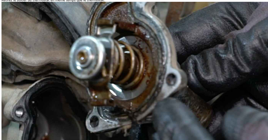
22 Couvrez l'emplacement de montage du boîtier du thermostat avec un chiffon en microfibre pour empêcher la saleté et les corps étrangers de pénétrer dans le système.
