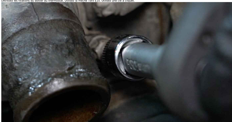
21 Retirez le boîtier du thermostat en même temps que le thermostat.
